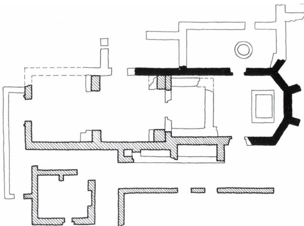
7. Veszprém, Szent Katalin domonkos apácazárda alaprajza. (Rhé Gyula munkája)
